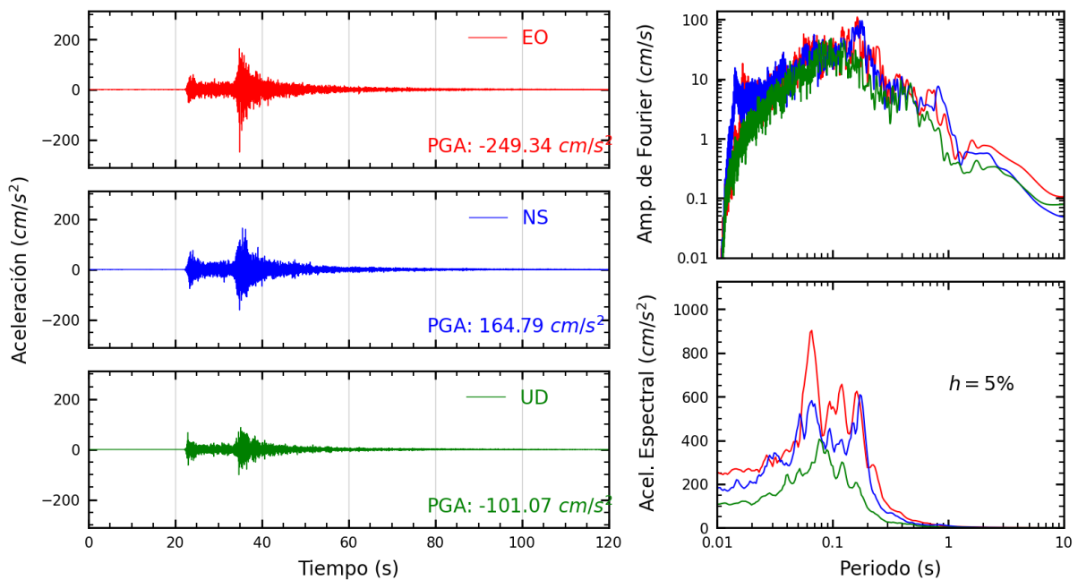
Figura A.26: Registros tiempo-historia, espectros de Fourier y de respuesta en las direcciones EO, NS y UD de la estación LIM028. Sismo de Lima, Lima - Lima de 2022-01-07, 05:27:05 (Hora local)
