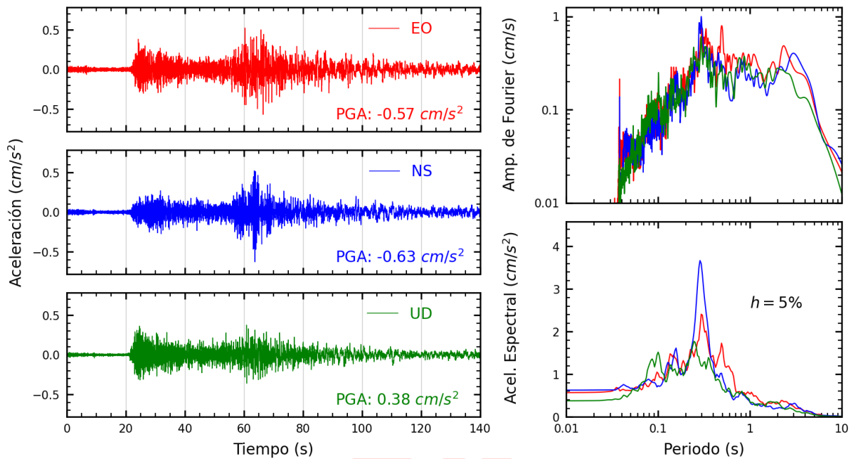
Figura A.1: Registros tiempo-historia, espectros de Fourier y de respuesta en las direcciones EO, NS y UD de la estación AYA001. Sismo de Lima, Lima - Lima de 2022-01-07, 05:27:05 (Hora local)
