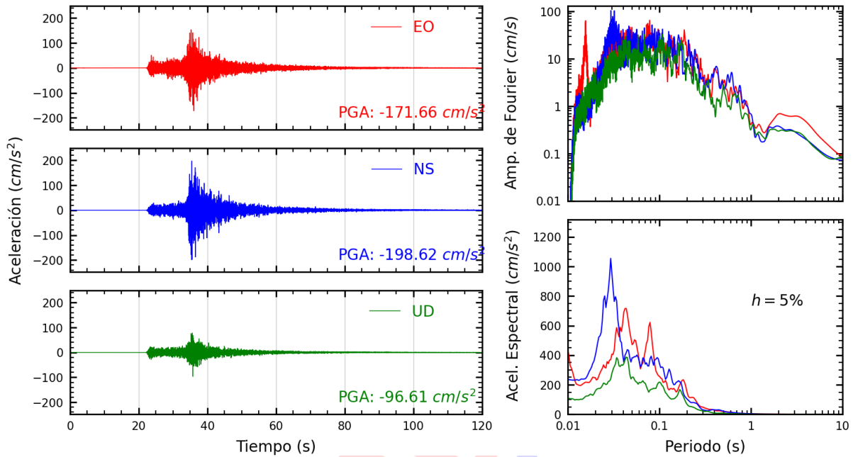
Figura A.23: Registros tiempo-historia, espectros de Fourier y de respuesta en las direcciones EO, NS y UD de la estación LIM024. Sismo de Lima, Lima - Lima de 2022-01-07, 05:27:05 (Hora local)
