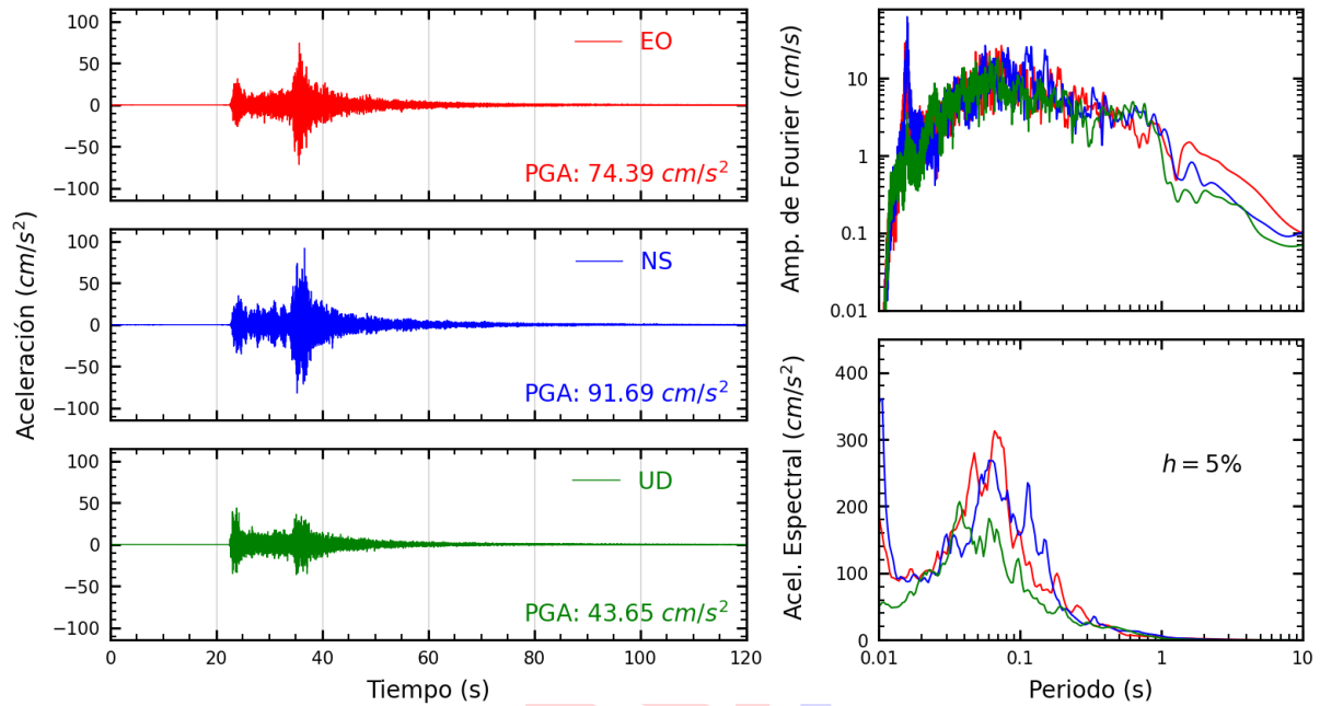
Figura A.17: Registros tiempo-historia, espectros de Fourier y de respuesta en las direcciones EO, NS y UD de la estación LIM014. Sismo de Lima, Lima - Lima de 2022-01-07, 05:27:05 (Hora local)
