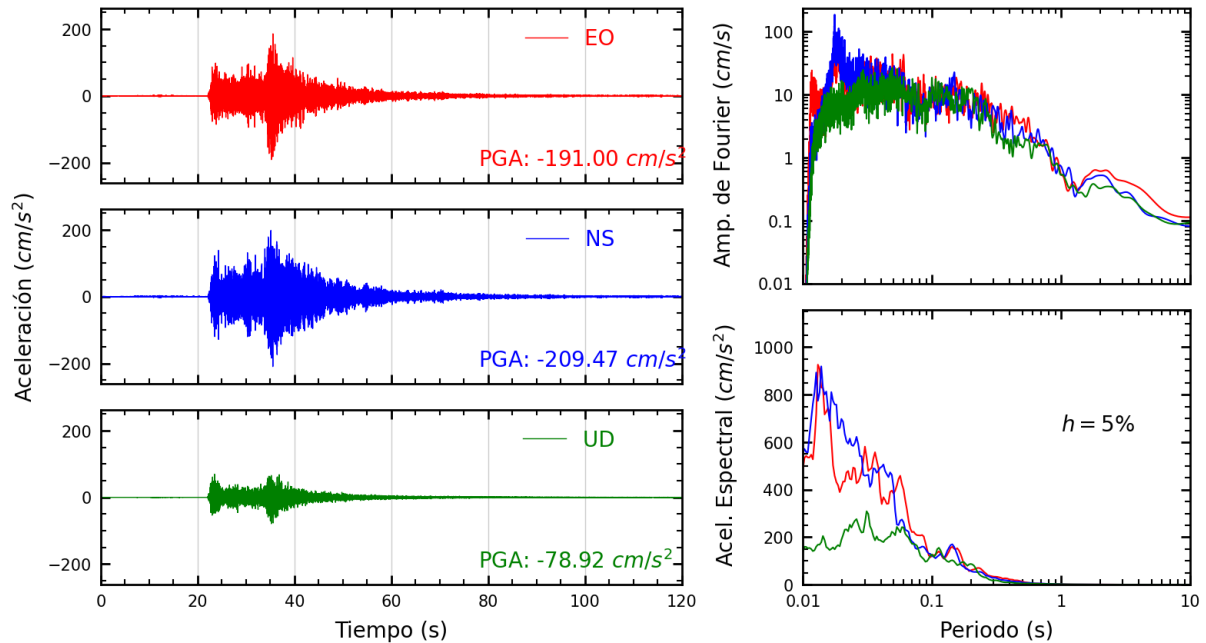
Figura A.15: Registros tiempo-historia, espectros de Fourier y de respuesta en las direcciones EO, NS y UD de la estación LIM010. Sismo de Lima, Lima - Lima de 2022-01-07, 05:27:05 (Hora local)
