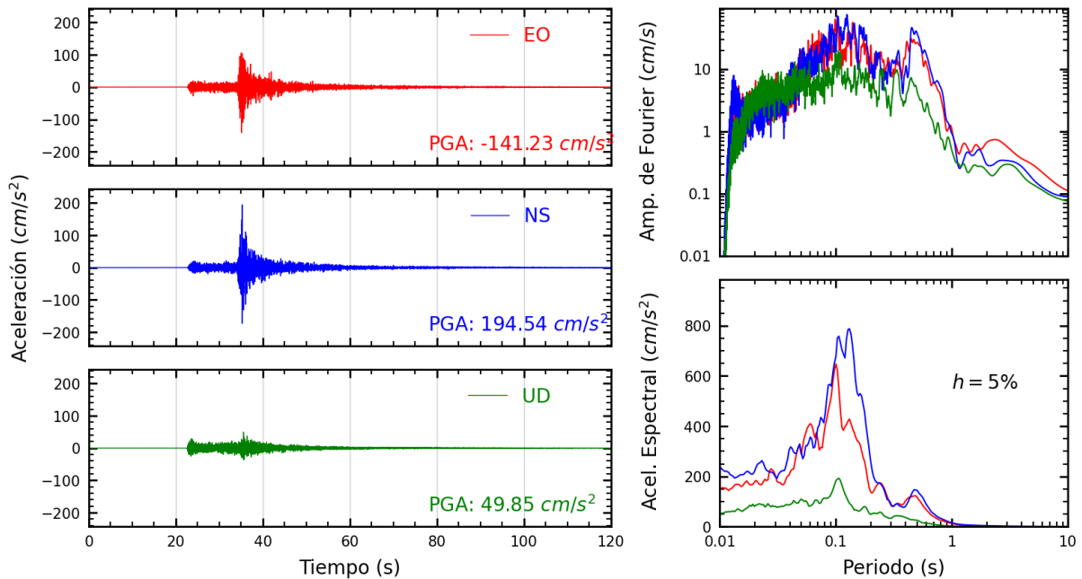
Figura A.10: Registros tiempo-historia, espectros de Fourier y de respuesta en las direcciones EO, NS y UD de la estación CAL012. Sismo de Lima, Lima - Lima de 2022-01-07, 05:27:05 (Hora local)
