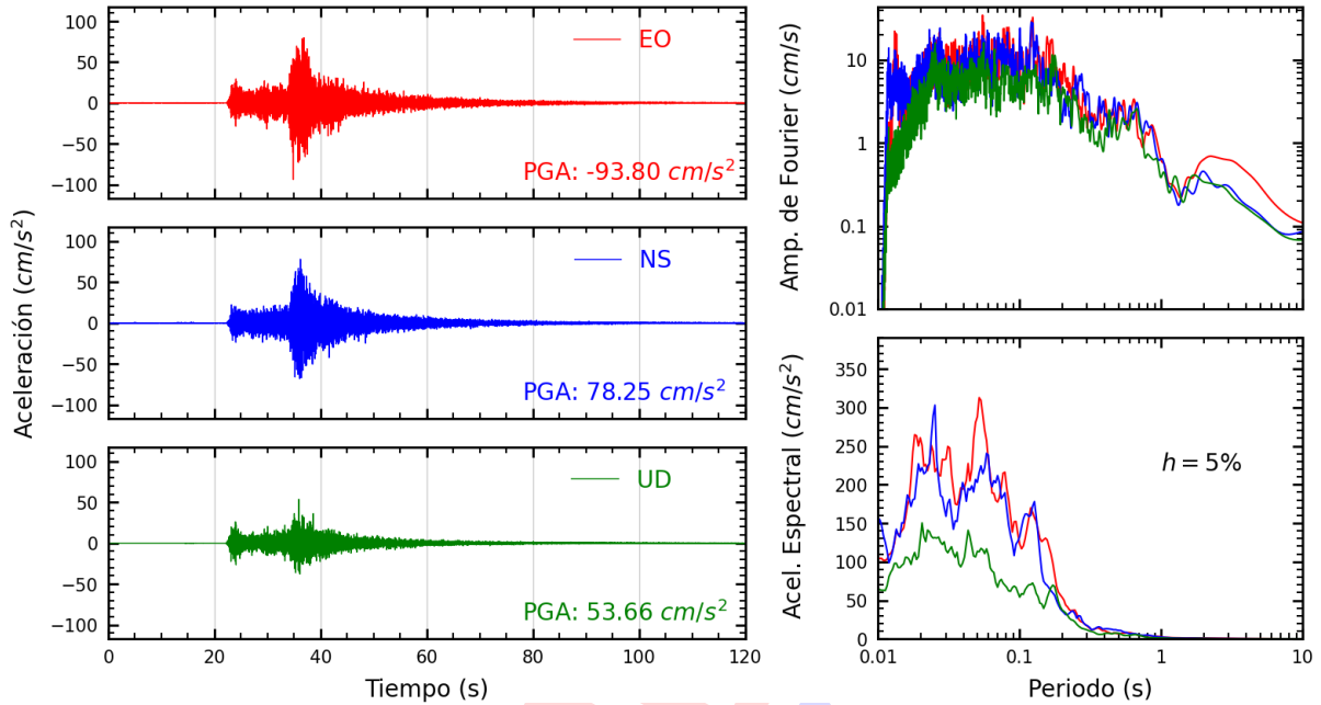
Figura A.13: Registros tiempo-historia, espectros de Fourier y de respuesta en las direcciones EO, NS y UD de la estación LIM002. Sismo de Lima, Lima - Lima de 2022-01-07, 05:27:05 (Hora local)
