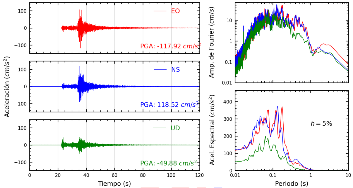
Figura A.29: Registros tiempo-historia, espectros de Fourier y de respuesta en las direcciones EO, NS y UD de la estación LIM032. Sismo de Lima, Lima - Lima de 2022-01-07, 05:27:05 (Hora local)
