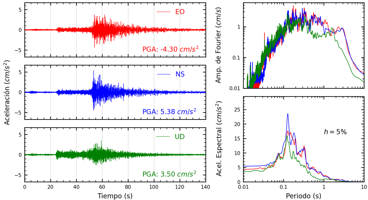
Figura A.11: Registros tiempo-historia, espectros de Fourier y de respuesta en las direcciones EO, NS y UD de la estación ICA003. Sismo de Lima, Lima - Lima de 2022-01-07, 05:27:05 (Hora local)
