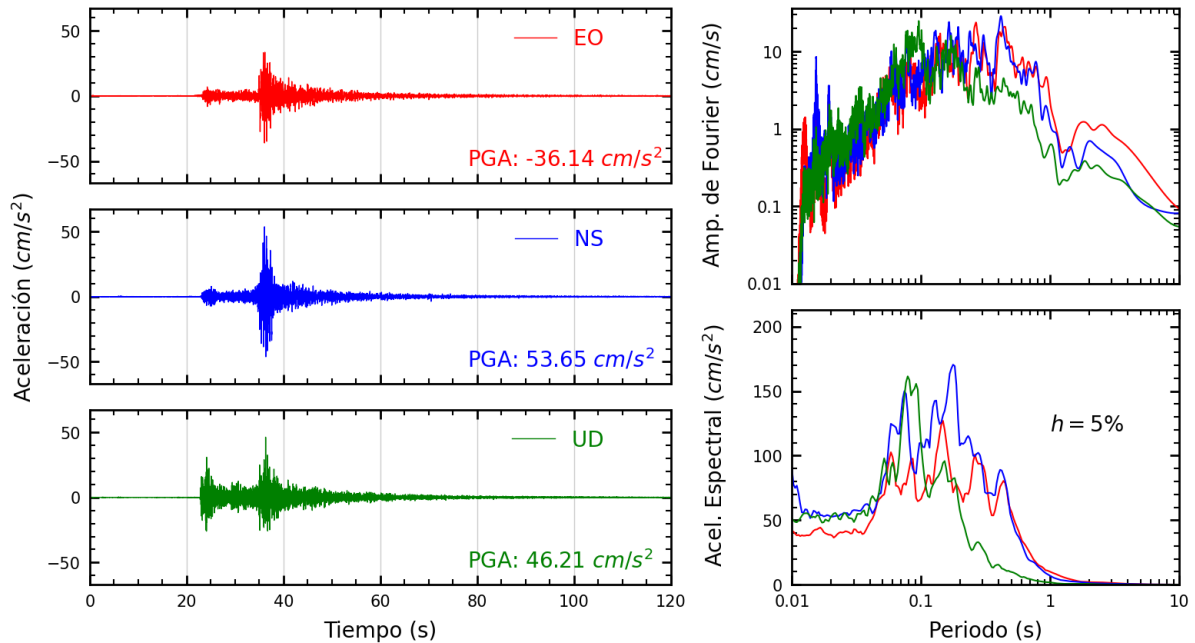
Figura A.5: Registros tiempo-historia, espectros de Fourier y de respuesta en las direcciones EO, NS y UD de la estación CAL004. Sismo de Lima, Lima - Lima de 2022-01-07, 05:27:05 (Hora local)
