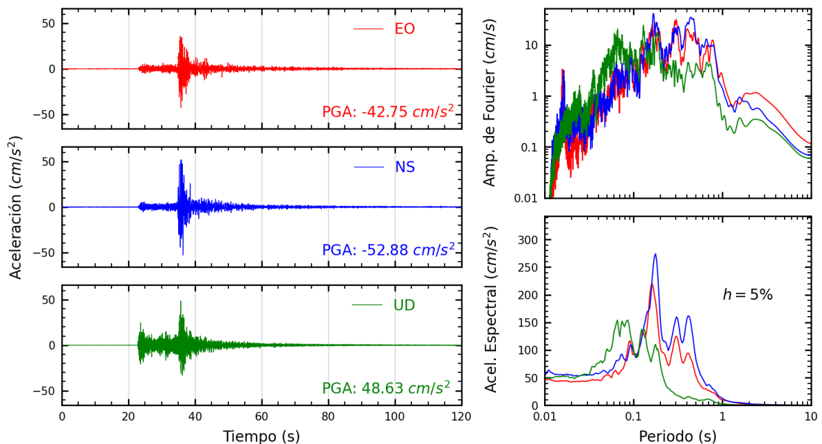
Figura A.6: Registros tiempo-historia, espectros de Fourier y de respuesta en las direcciones EO, NS y UD de la estación CAL005. Sismo de Lima, Lima - Lima de 2022-01-07, 05:27:05 (Hora local)
