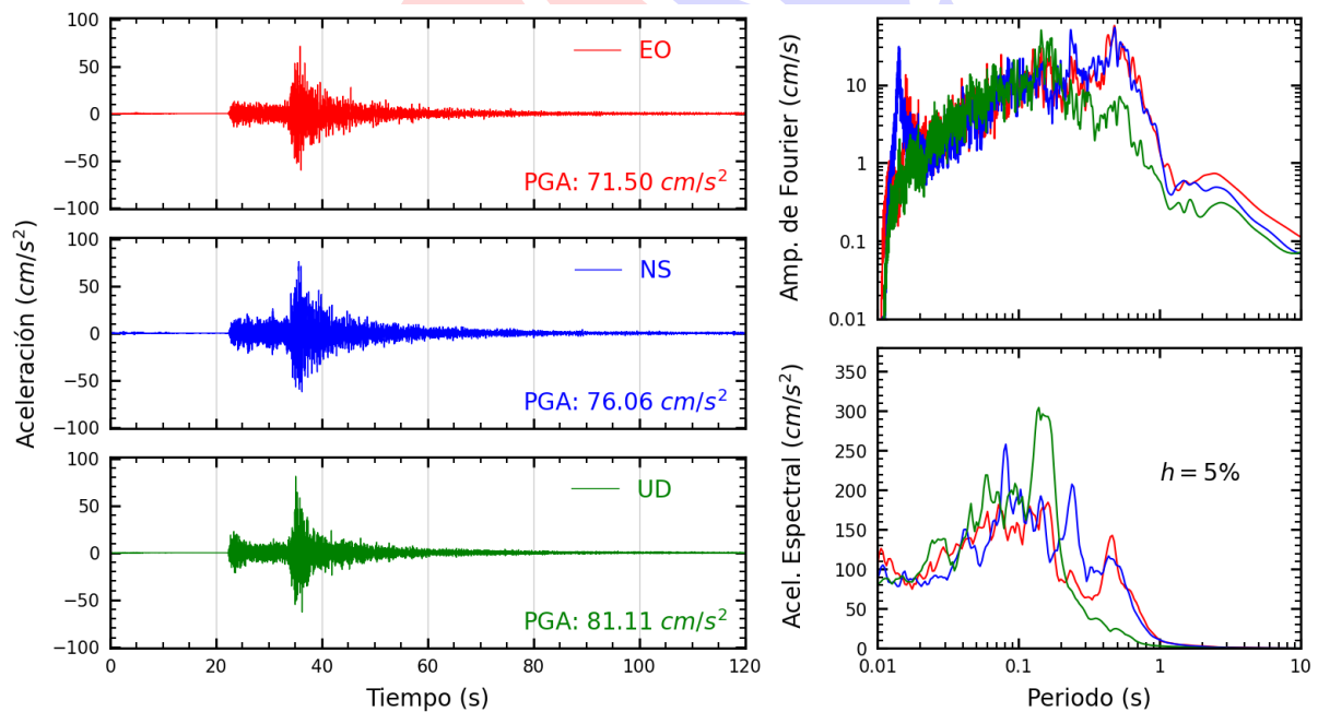
Figura A.22: Registros tiempo-historia, espectros de Fourier y de respuesta en las direcciones EO, NS y UD de la estación LIM022. Sismo de Lima, Lima - Lima de 2022-01-07, 05:27:05 (Hora local)
