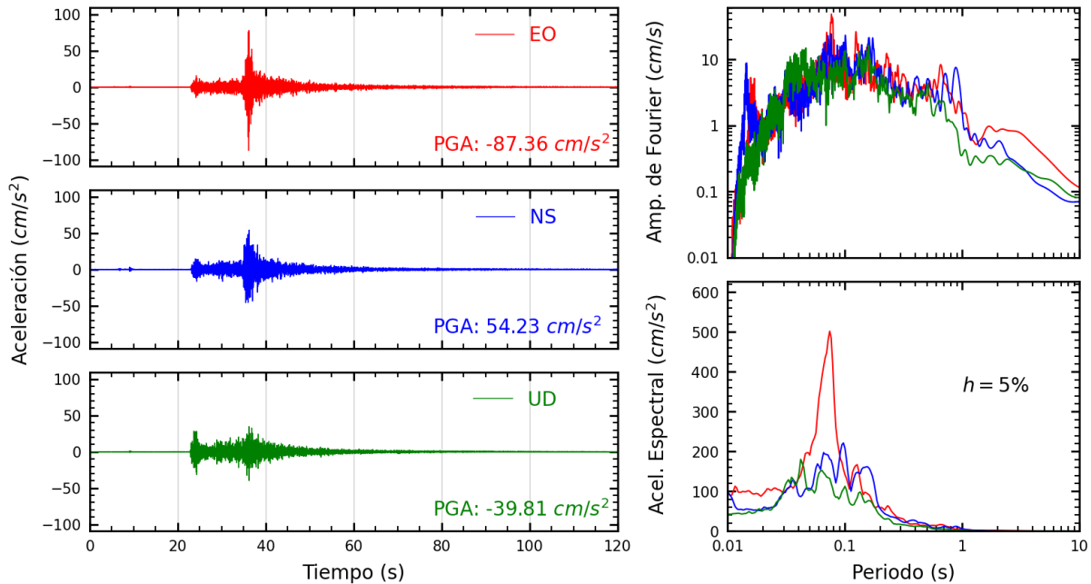
Figura A.27: Registros tiempo-historia, espectros de Fourier y de respuesta en las direcciones EO, NS y UD de la estación LIM029. Sismo de Lima, Lima - Lima de 2022-01-07, 05:27:05 (Hora local)
