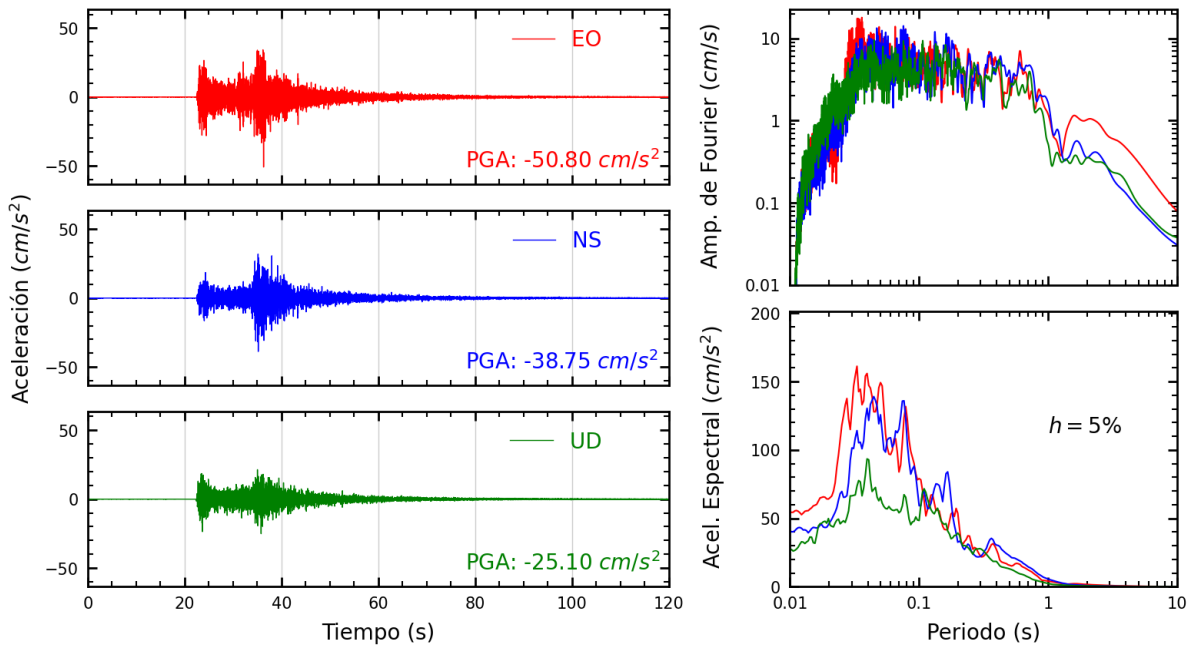
Figura A.14: Registros tiempo-historia, espectros de Fourier y de respuesta en las direcciones EO, NS y UD de la estación LIM009. Sismo de Lima, Lima - Lima de 2022-01-07, 05:27:05 (Hora local)
