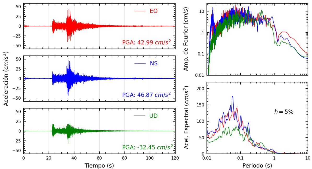
Figura A.18: Registros tiempo-historia, espectros de Fourier y de respuesta en las direcciones EO, NS y UD de la estación LIM015. Sismo de Lima, Lima - Lima de 2022-01-07, 05:27:05 (Hora local)
