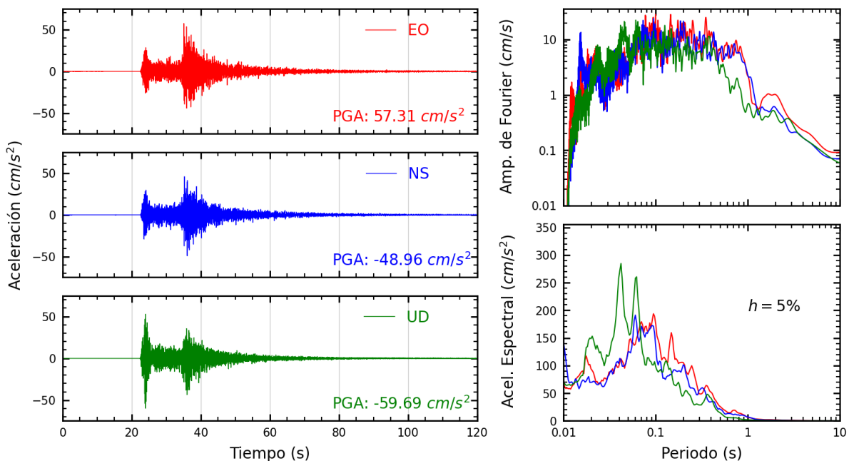
Figura A.28: Registros tiempo-historia, espectros de Fourier y de respuesta en las direcciones EO, NS y UD de la estación LIM030. Sismo de Lima, Lima - Lima de 2022-01-07, 05:27:05 (Hora local)
