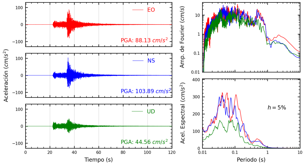
Figura A.20: Registros tiempo-historia, espectros de Fourier y de respuesta en las direcciones EO, NS y UD de la estación LIM019. Sismo de Lima, Lima - Lima de 2022-01-07, 05:27:05 (Hora local)
