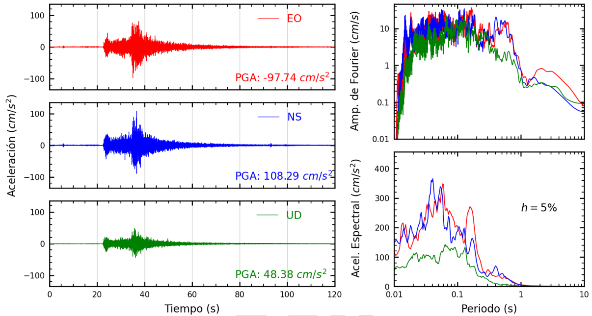
Figura A.19: Registros tiempo-historia, espectros de Fourier y de respuesta en las direcciones EO, NS y UD de la estación LIM018. Sismo de Lima, Lima - Lima de 2022-01-07, 05:27:05 (Hora local)
