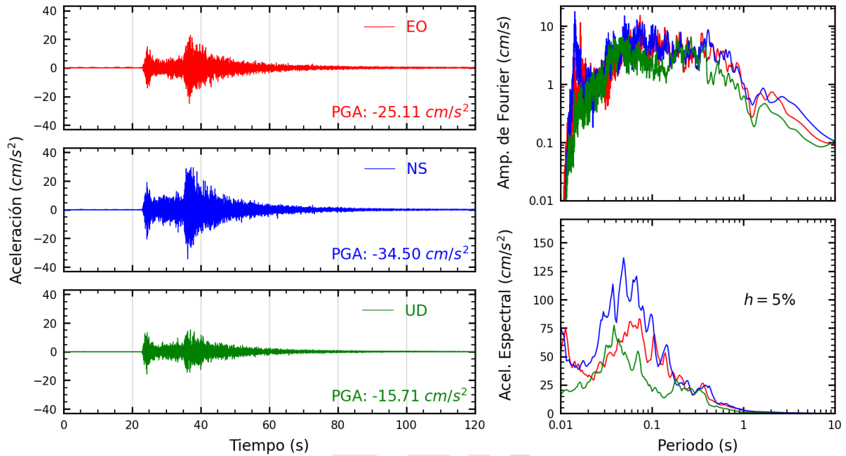
Figura A.25: Registros tiempo-historia, espectros de Fourier y de respuesta en las direcciones EO, NS y UD de la estación LIM027. Sismo de Lima, Lima - Lima de 2022-01-07, 05:27:05 (Hora local)
