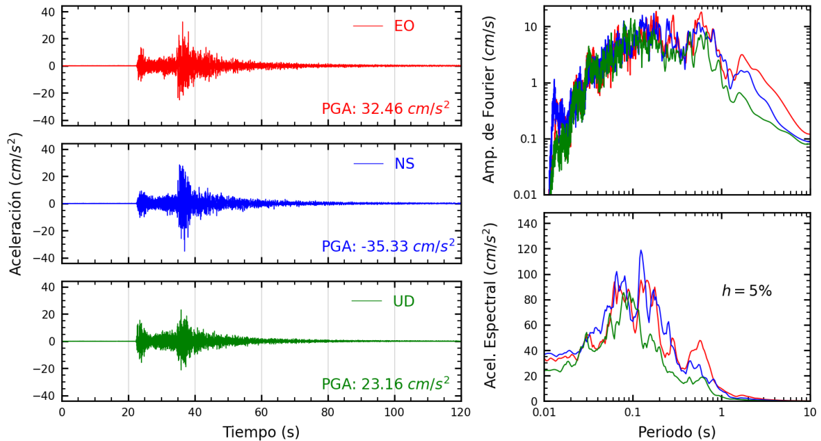
Figura A.3: Registros tiempo-historia, espectros de Fourier y de respuesta en las direcciones EO, NS y UD de la estación CAL002. Sismo de Lima, Lima - Lima de 2022-01-07, 05:27:05 (Hora local)
