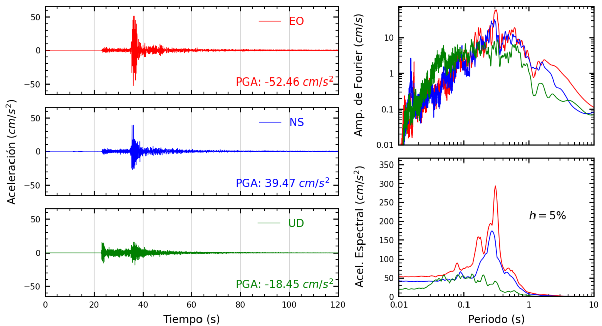
Figura A.4: Registros tiempo-historia, espectros de Fourier y de respuesta en las direcciones EO, NS y UD de la estación CAL003. Sismo de Lima, Lima - Lima de 2022-01-07, 05:27:05 (Hora local)
