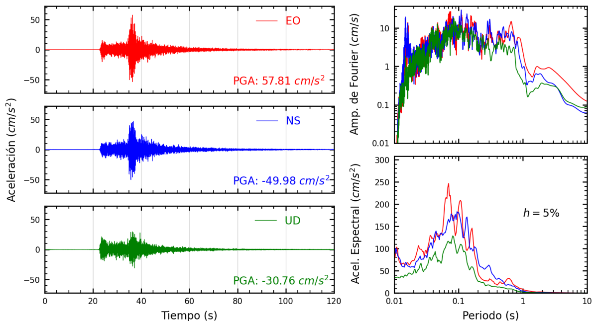
Figura A.8: Registros tiempo-historia, espectros de Fourier y de respuesta en las direcciones EO, NS y UD de la estación CAL007. Sismo de Lima, Lima - Lima de 2022-01-07, 05:27:05 (Hora local)
