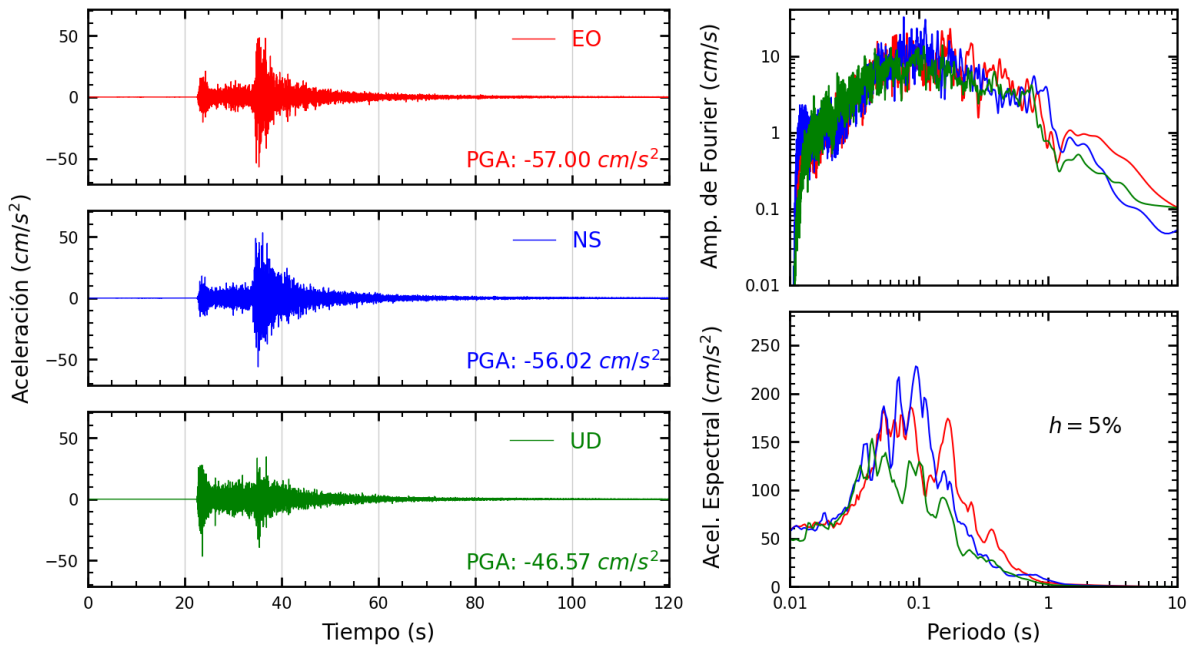
Figura A.24: Registros tiempo-historia, espectros de Fourier y de respuesta en las direcciones EO, NS y UD de la estación LIM026. Sismo de Lima, Lima - Lima de 2022-01-07, 05:27:05 (Hora local)
