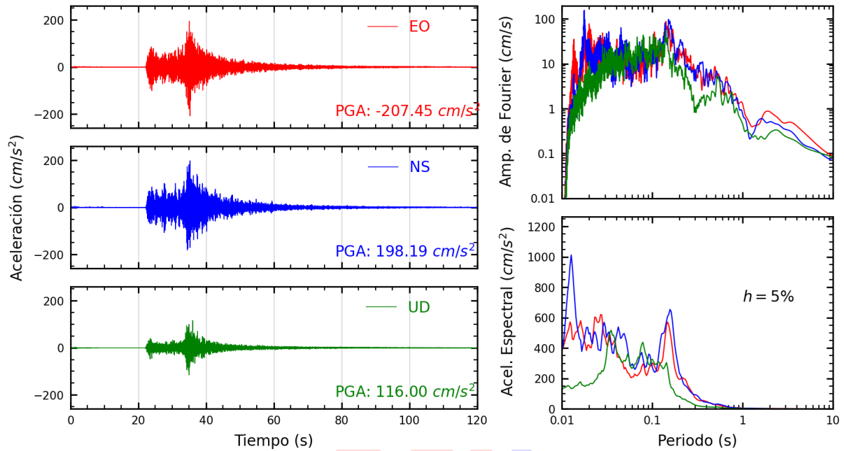
Figura A.21: Registros tiempo-historia, espectros de Fourier y de respuesta en las direcciones EO, NS y UD de la estación LIM021. Sismo de Lima, Lima - Lima de 2022-01-07, 05:27:05 (Hora local)
