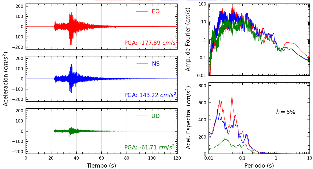
Figura A.12: Registros tiempo-historia, espectros de Fourier y de respuesta en las direcciones EO, NS y UD de la estación LIM001. Sismo de Lima, Lima - Lima de 2022-01-07, 05:27:05 (Hora local)
