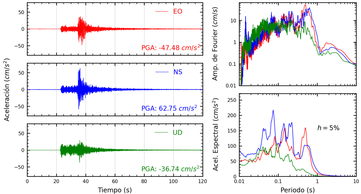
Figura A.7: Registros tiempo-historia, espectros de Fourier y de respuesta en las direcciones EO, NS y UD de la estación CAL006. Sismo de Lima, Lima - Lima de 2022-01-07, 05:27:05 (Hora local)
