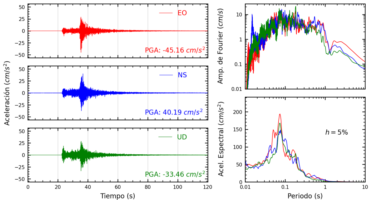
Figura A.16: Registros tiempo-historia, espectros de Fourier y de respuesta en las direcciones EO, NS y UD de la estación LIM012. Sismo de Lima, Lima - Lima de 2022-01-07, 05:27:05 (Hora local)
