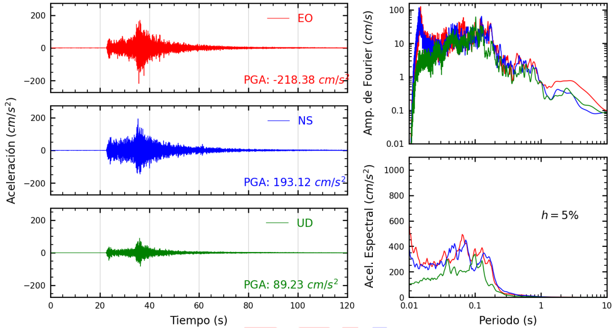
Figura A.9: Registros tiempo-historia, espectros de Fourier y de respuesta en las direcciones EO, NS y UD de la estación CAL008. Sismo de Lima, Lima - Lima de 2022-01-07, 05:27:05 (Hora local)
