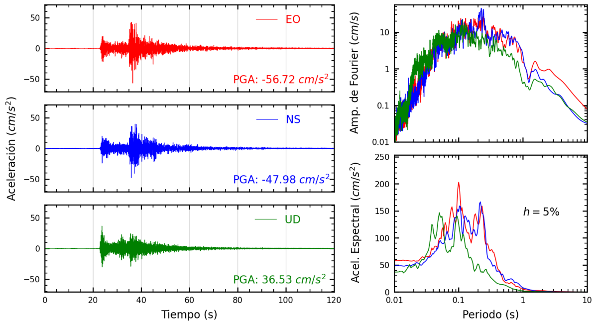
Figura A.30: Registros tiempo-historia, espectros de Fourier y de respuesta en las direcciones EO, NS y UD de la estación LIM033. Sismo de Lima, Lima - Lima de 2022-01-07, 05:27:05 (Hora local)
