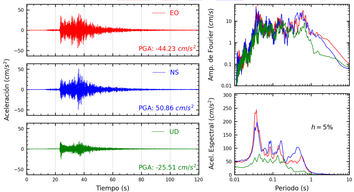
Figura A.2: Registros tiempo-historia, espectros de Fourier y de respuesta en las direcciones EO, NS y UD de la estación CAL001. Sismo de Lima, Lima - Lima de 2022-01-07, 05:27:05 (Hora local)
